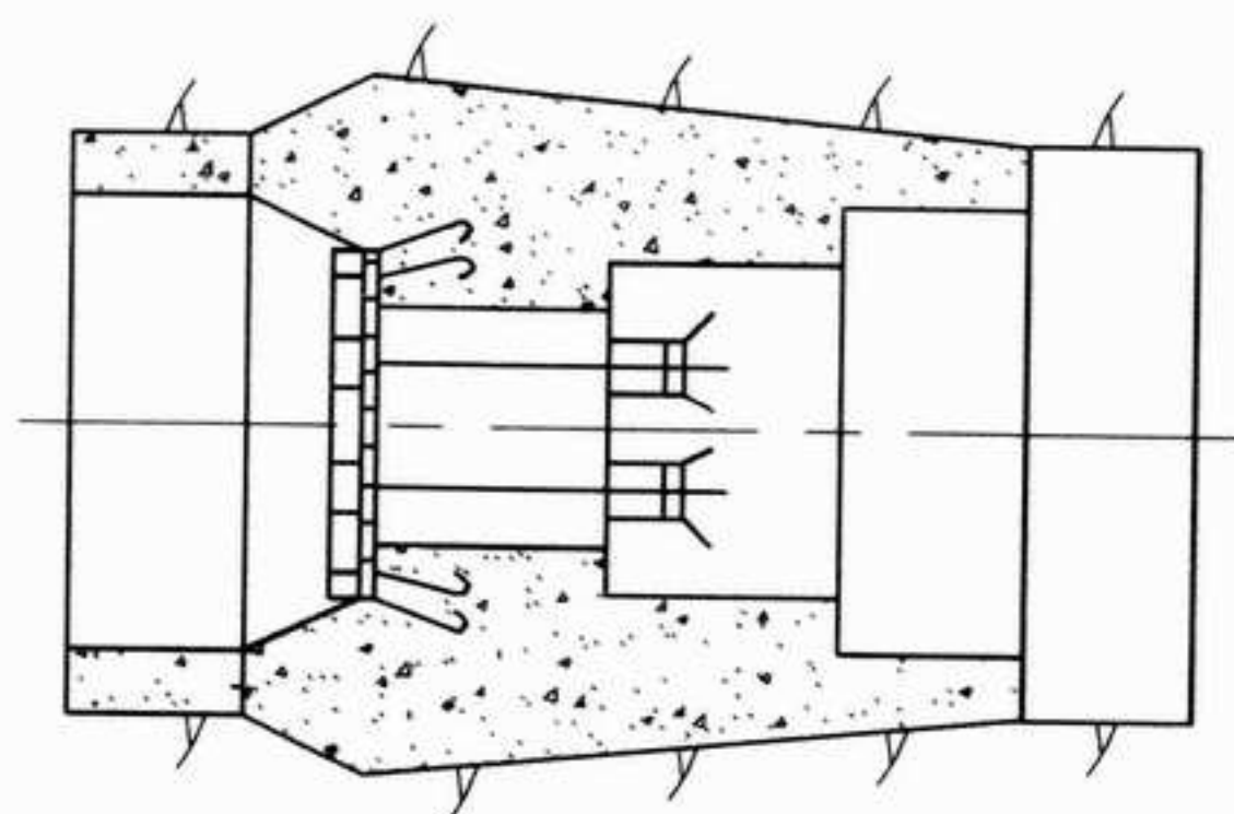
(a) 塞形堵头
