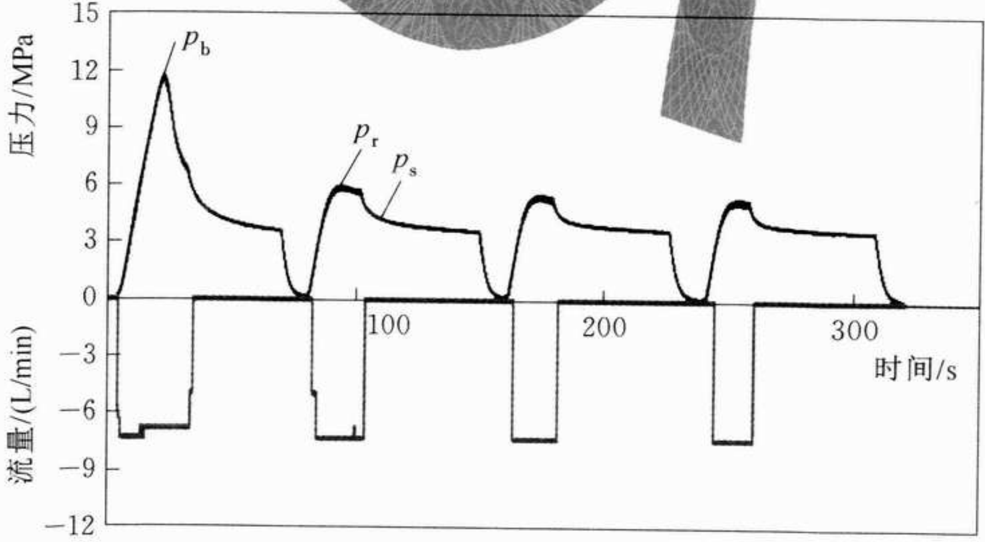
图 14 水压致裂压力—时间过程曲线
