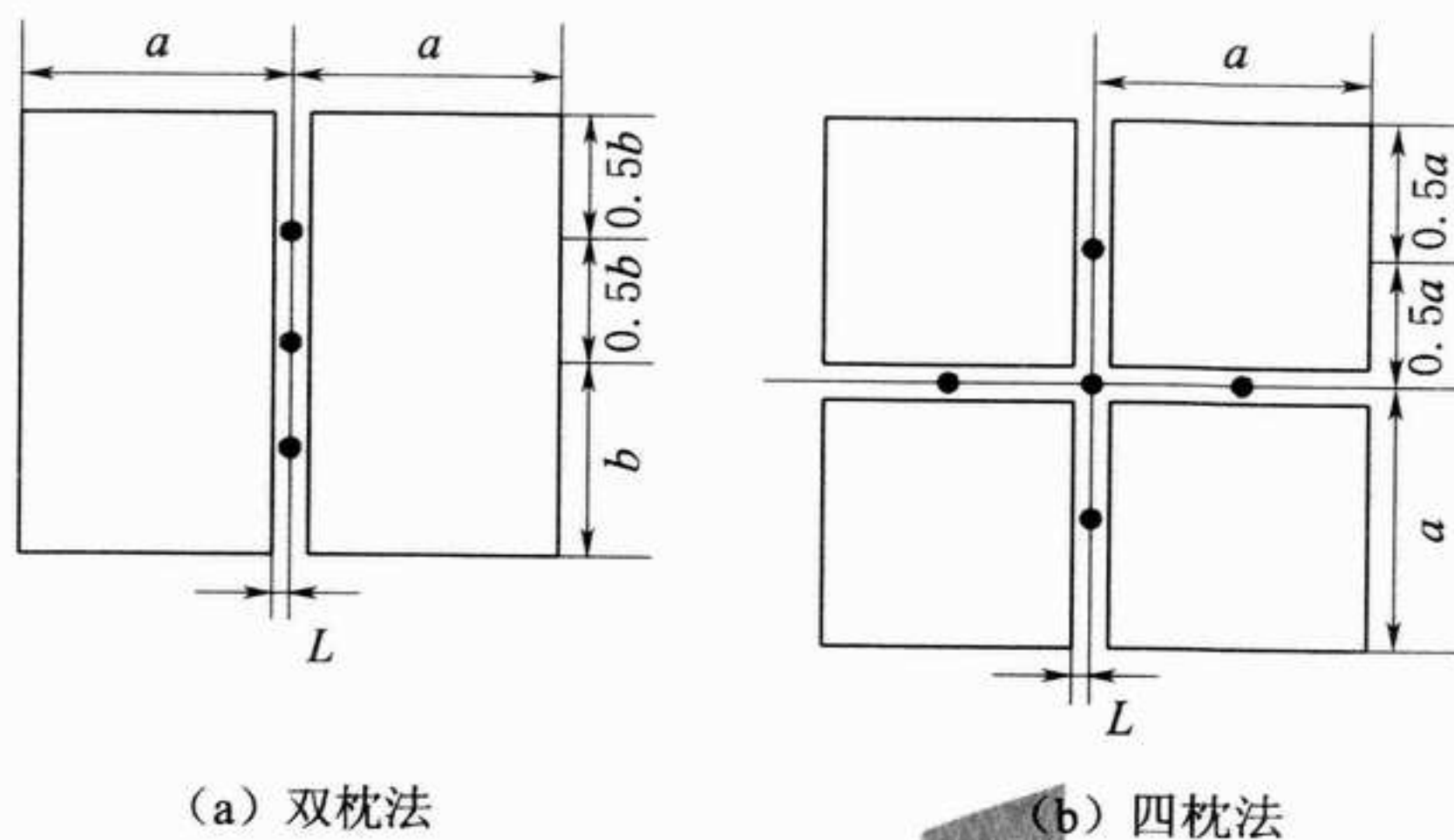
图 6.1.8 柔性承压板法测表布置示意图
