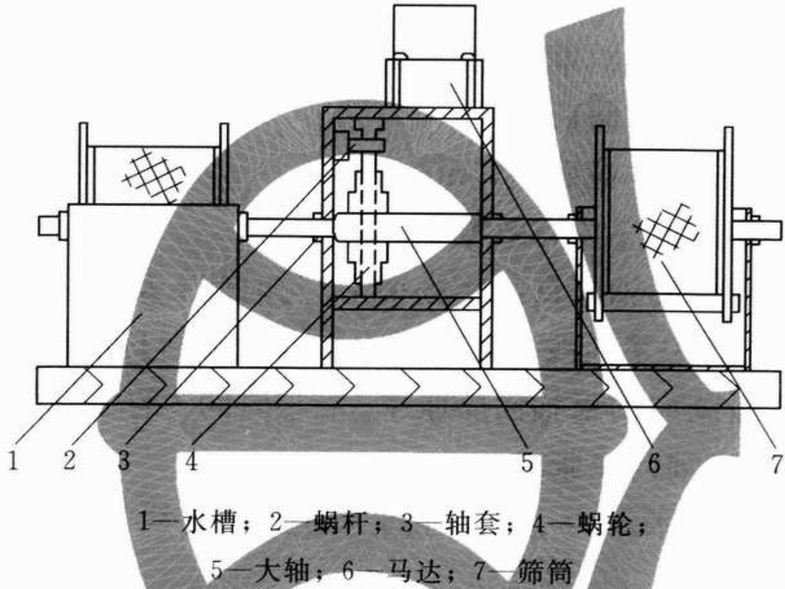
图 4.6.4 耐崩解性试验仪示意图
