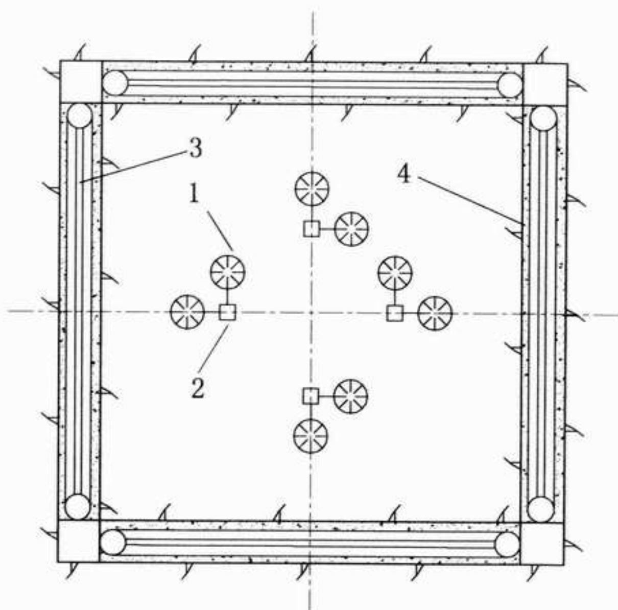
1—测表；2—标点；3—液压枕；4—砂浆
