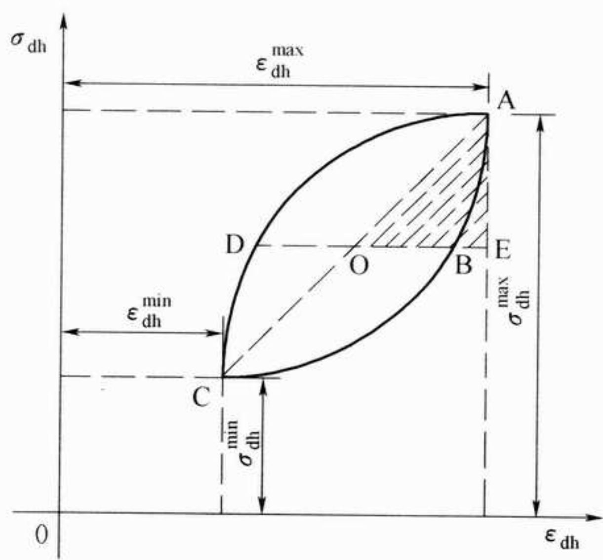
图 5.9.8-1 应力应变滞回圈
