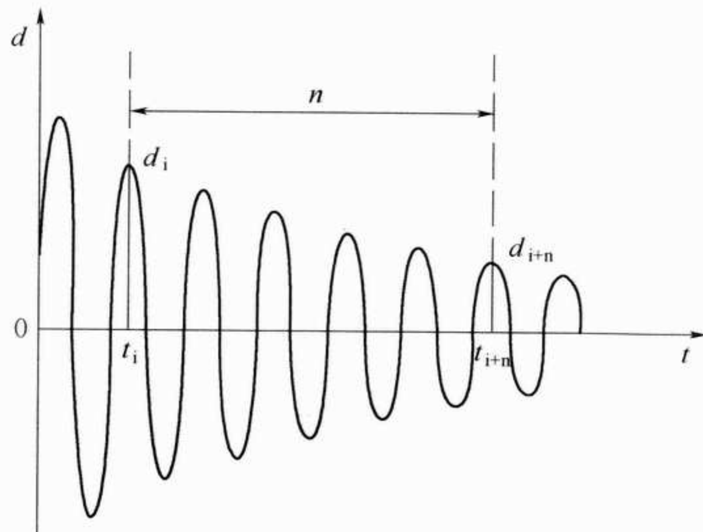
图 5.9.9 振幅随时间的衰减关系曲线
