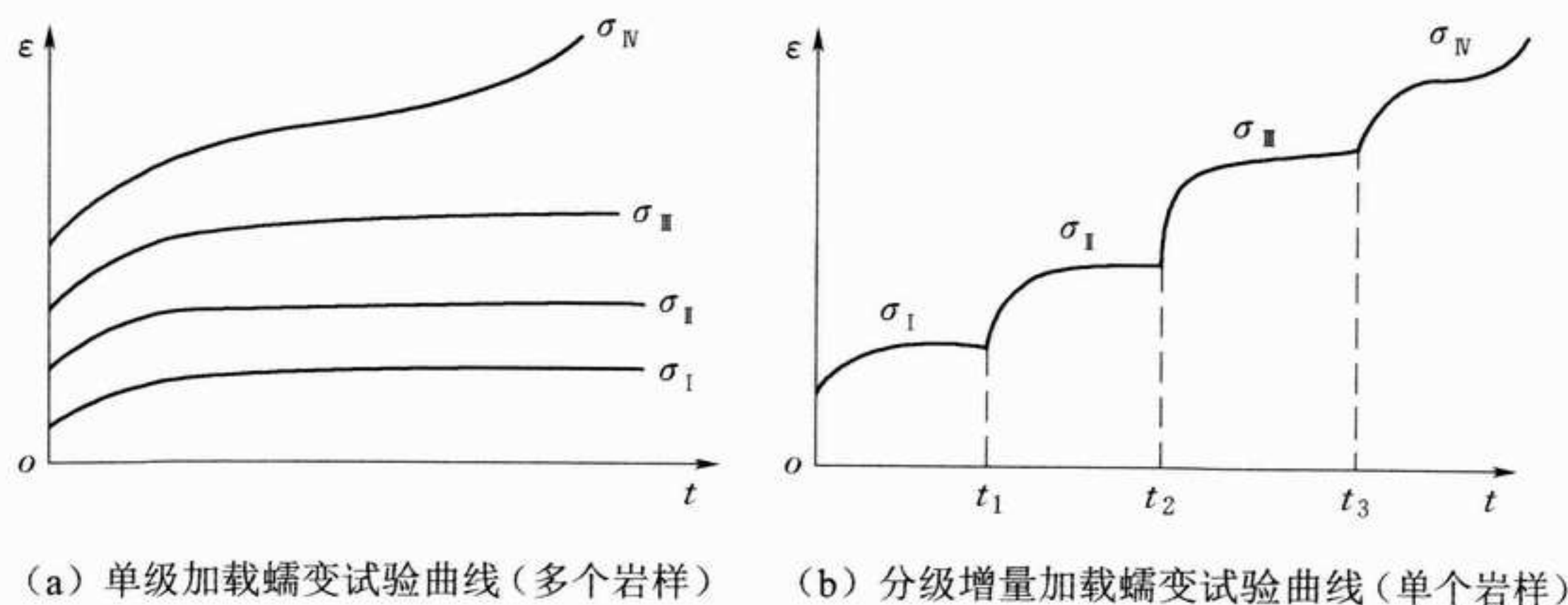
图 11 单轴压缩蠕变试验中的单级加载和分级加载方式
