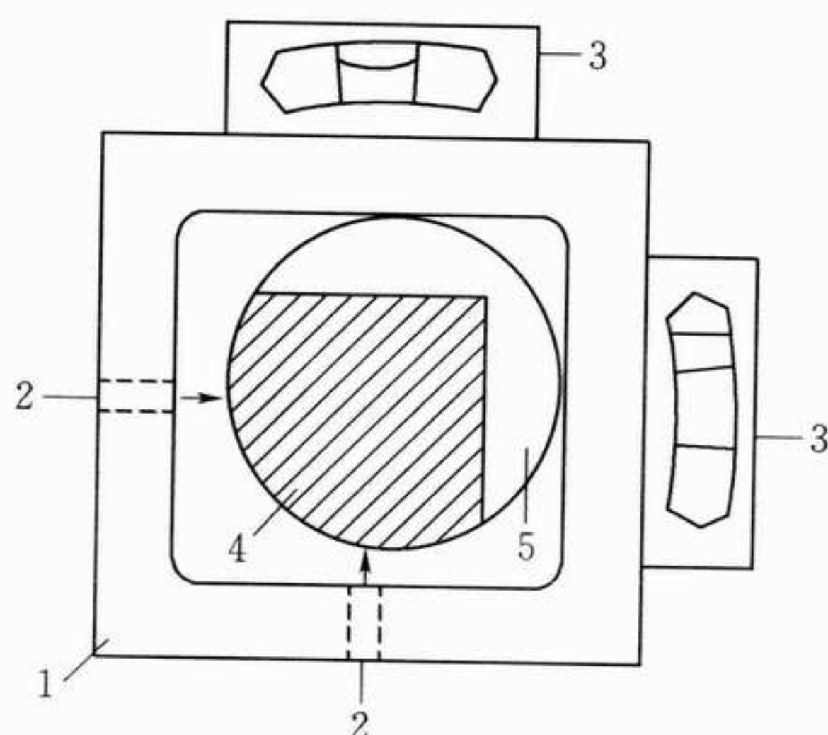
1—金属框架；2—紧固螺杆；3—水准仪；4—试件；5—切口
