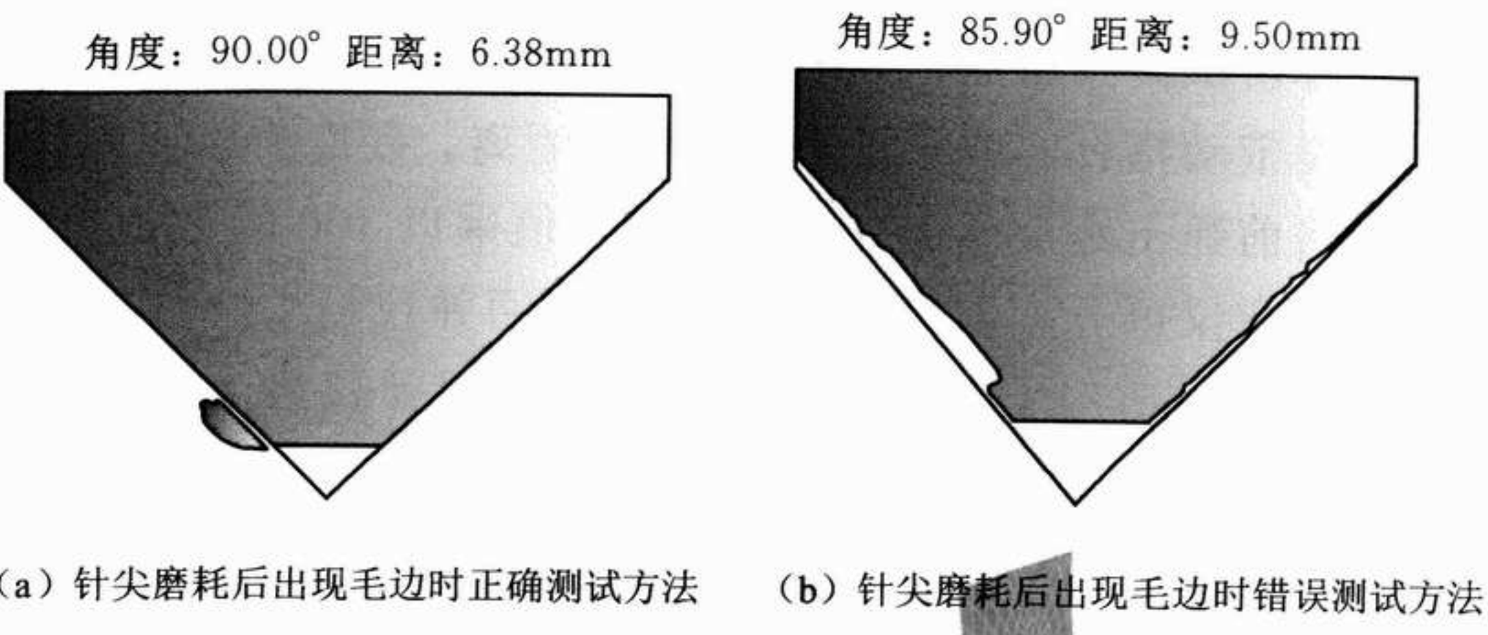
图 2 针尖磨损侧视图
