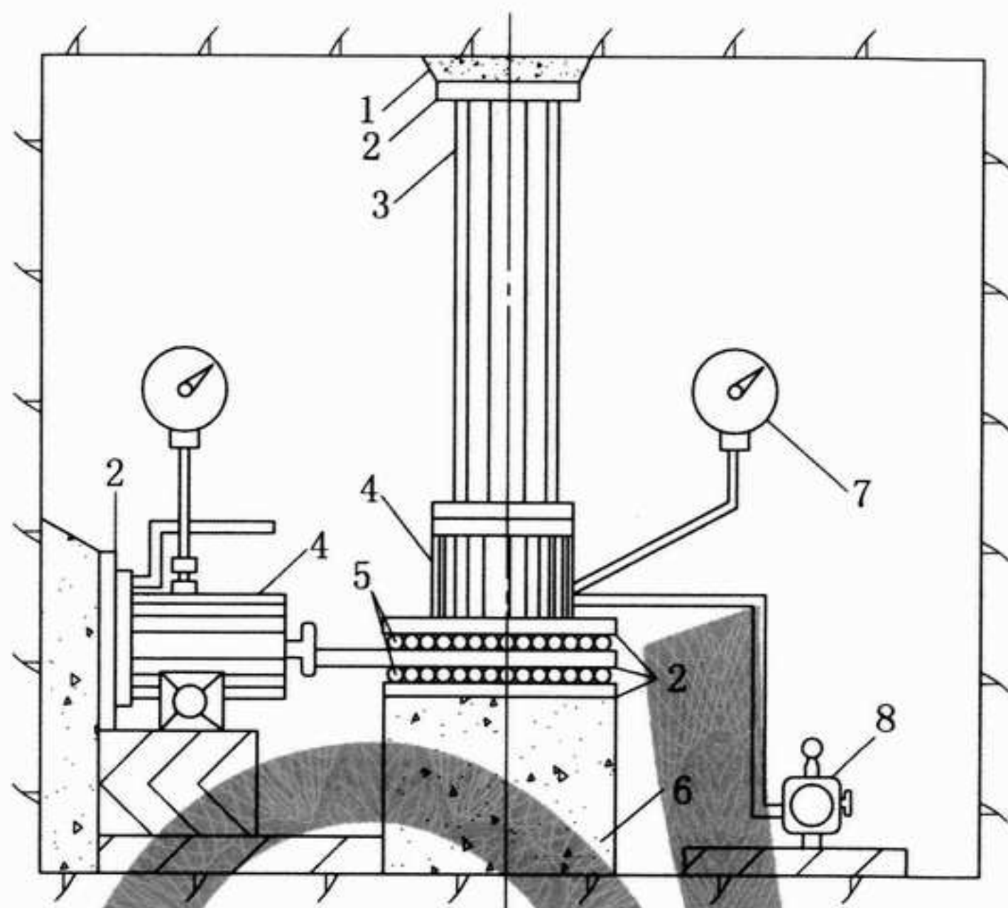
1—砂浆顶板；2—钢垫板；3—传力柱；4—液压千斤顶； 5—滚轴排；6—混凝土平台；7—压力表；8—液压泵
