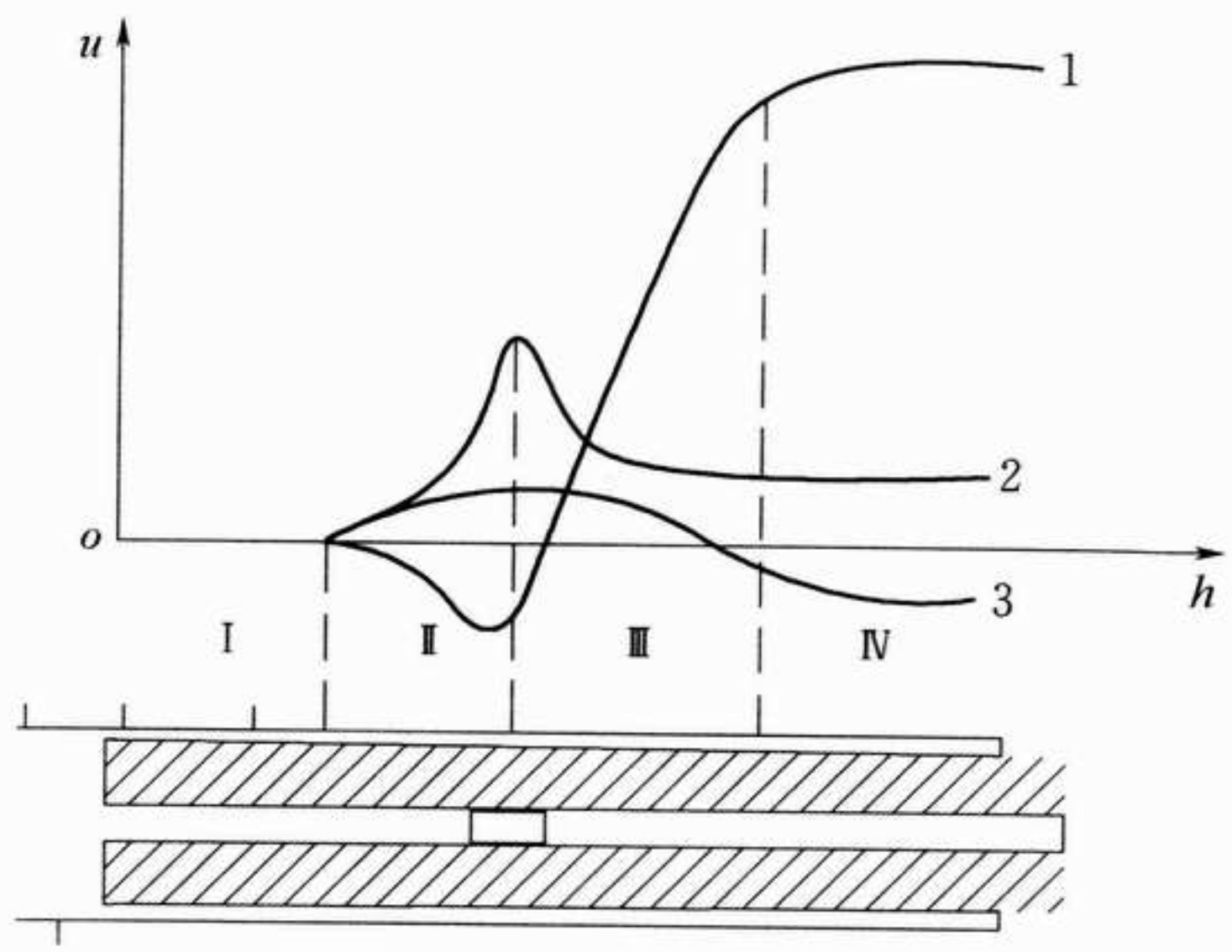
I—无应力影响区，解除时无变化；II—应力集中区，由于施钻引起的应力集中；III—应力释放区，随着解除过程应力的变化； IV—应变稳定区，应变值随解除深度加深逐渐趋于稳定
