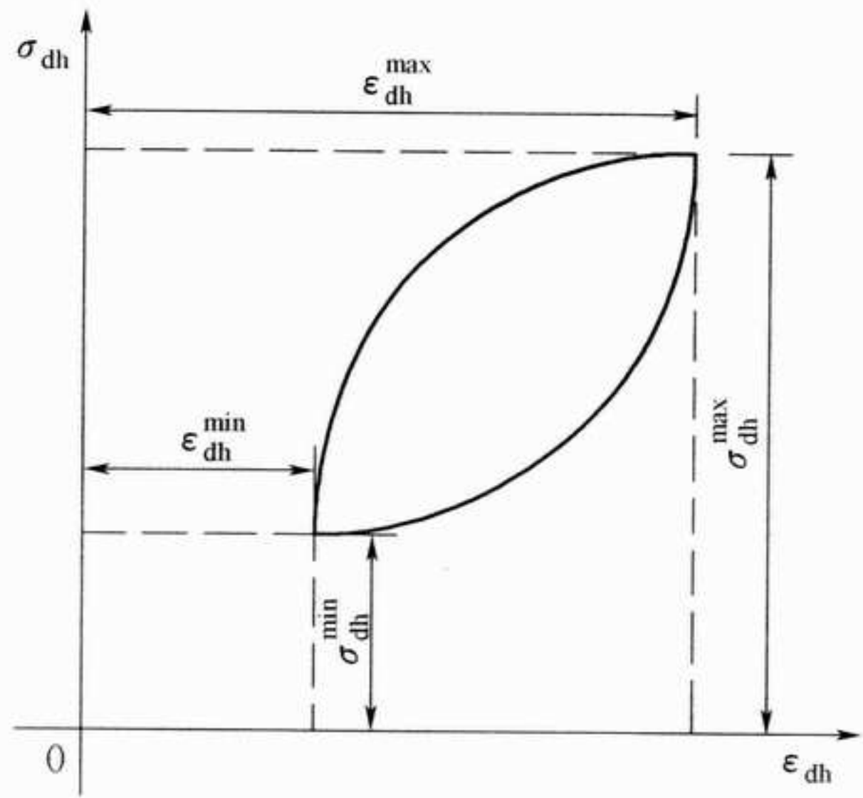
图 5.8.9 应力应变滞回圈
