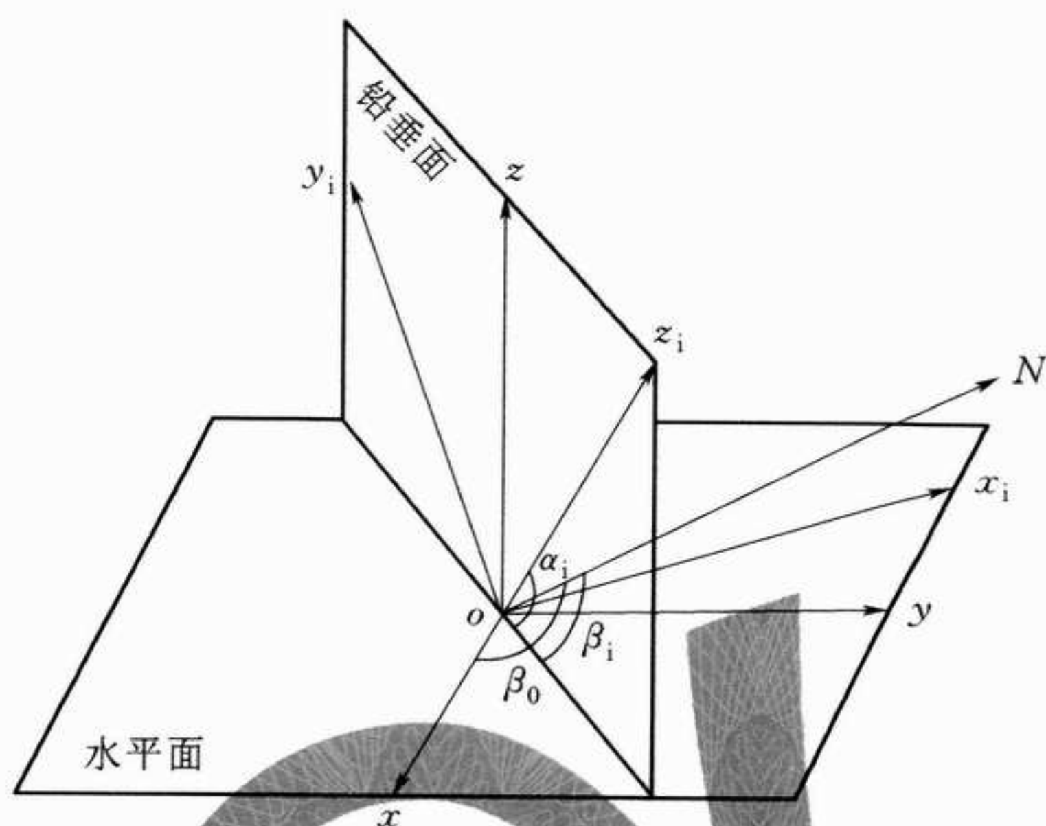
图 G. 2. 3 钻孔坐标系与大地坐标系相互关系
