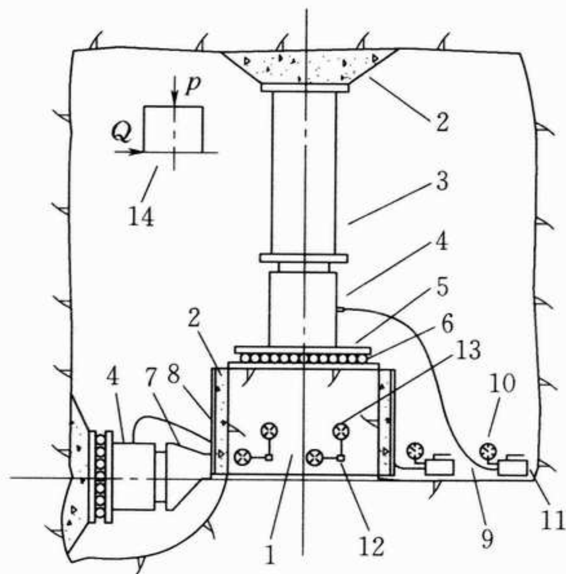
1—试体；2—砂浆；3—传力柱；4—液压千斤顶；5—钢垫板；6—滚轴排； 7—传力箱；8—钢模；9—液压管路；10—压力表；11—液压泵； 12—测量标点；13—位移测表；14—受力简图
