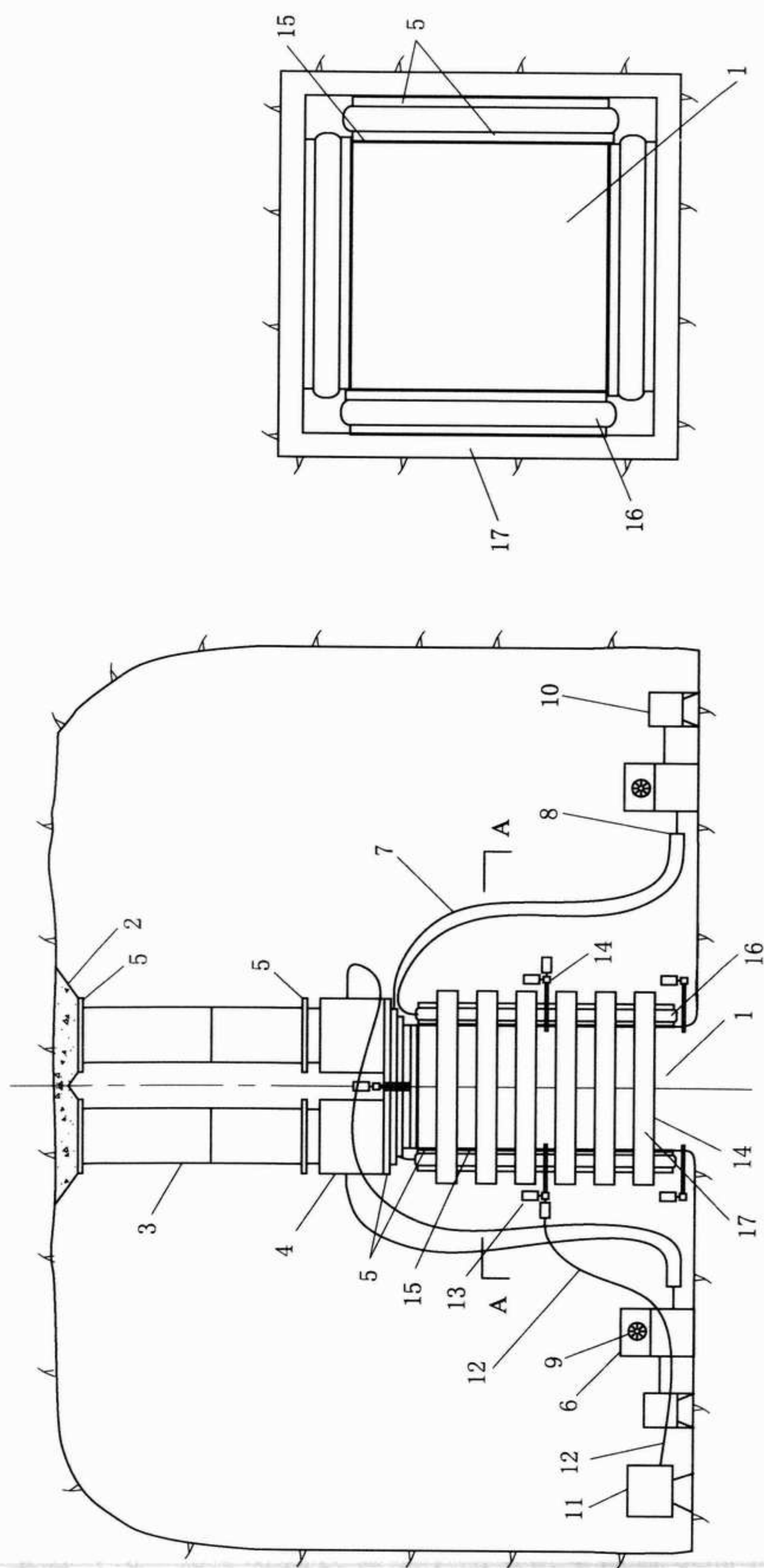
(a) 立视图
